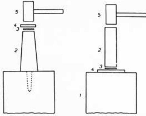
5. Försök till rekonstruktion av brakteatpräglingens metod, till vänster med en fixerad konisk understamp, till höger med lös cylindrisk överstamp som man tror använts i Lödöse. Myntämnet (silverplåten) lades på ett mjukt underlag av läder eller bly.
